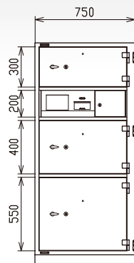
MH-02 (扉式) オープン価格(受注生産) 外寸 W750×D600×H1650
