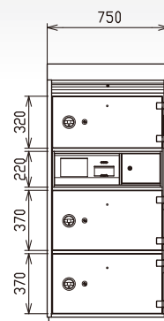
MH-03 (シャッター式) オープン価格(受注生産) 外寸 W750×D600×H1600
